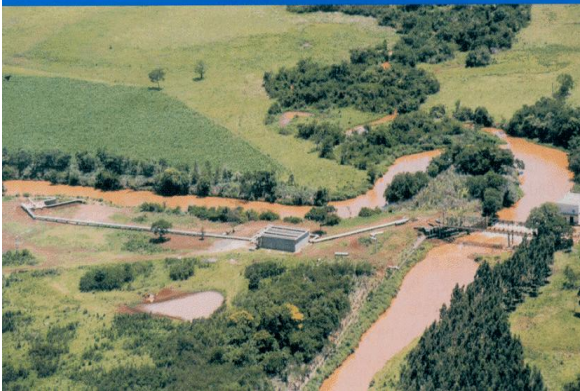
FIGURA 6 - VISTA AÉREA DOS RIOS PIRAPÓ E SARANDI - CAPTAÇÃO DA SANEPAR EM MARINGÁ
